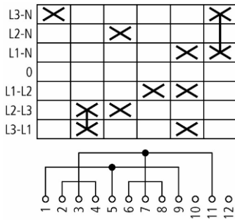
Šematski prikaz
