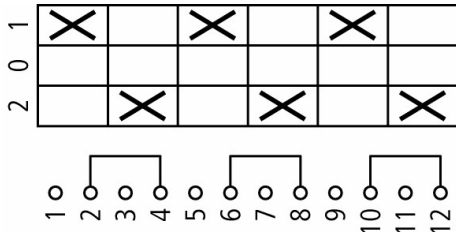
Šematski prikaz
