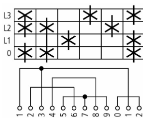
Šematski prikaz
