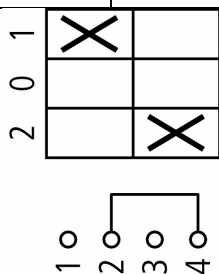
Šematski prikaz
