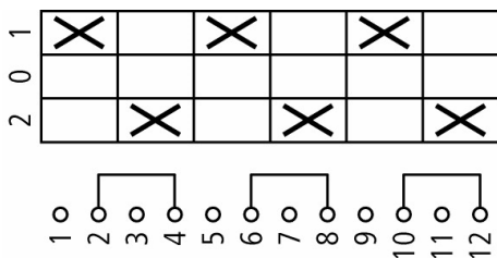
Šematski prikaz
